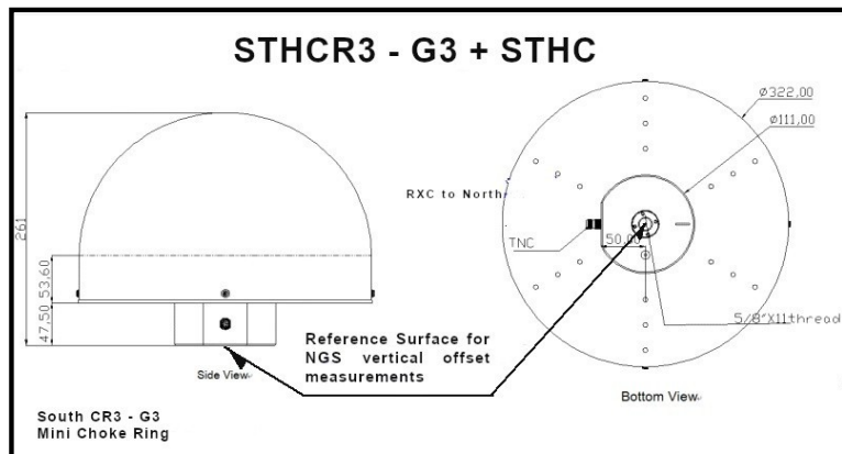
Croquis Antena Altura ARP = 0.0000
